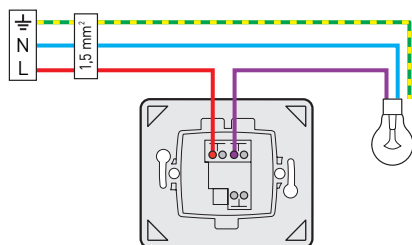
INTERRUPTEUR SANS VOYANT
