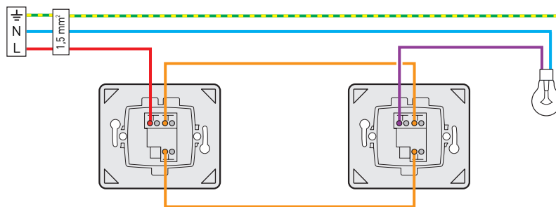
VA-ET-VIENT AVEC VOYANT LUMINEUX
