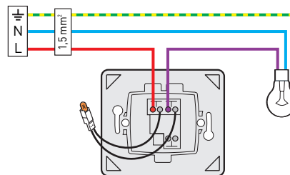
INTERRUPTEUR AVEC VOYANT LUMINEUX
